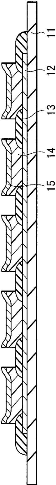
FIG. 6B
